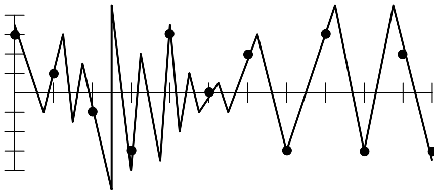
Рис. 7. Оцифрованный (точки) аналоговый (непрерывная кривая) звук. Горизонтальная ось обозначает время, вертикальная — амплитуду звука. Рисками на осях обозначены точки дискретизации звука
