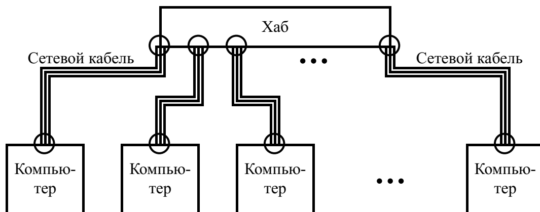
Рис. 2. Звездообразная архитектура сети. Кругами обведены разъемы
